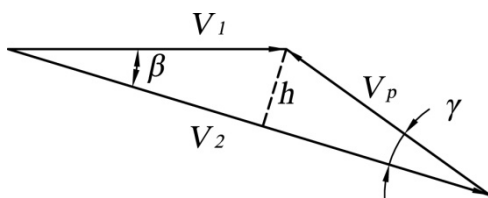
Рис. 2. План швидкостей
