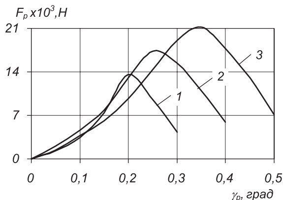
Рис. 3. Графіки залежності сил різання від глибини різання ножа в картон завтовшки: \Delta = 0,3 \text{ мм} (1); 0,4 \text{ мм} (2); 0,5 \text{ мм} (3)
